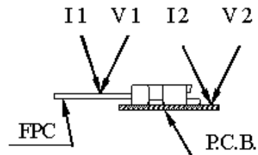
図 1. 接触抵抗測定方法
